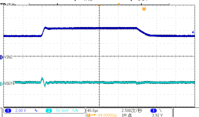
AVDD2, V_{IN2}=3.3\sim 4.5V , I_{OUT}=1mA
