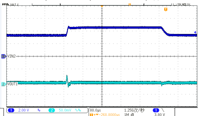
DVDD1, V_{IN1}=1.35V , V_{IN2}=3.3\sim 4.5V , I_{OUT}=1mA
