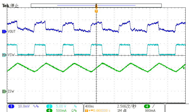
Ripple : VIN=5V, VO=1.8V, EN=3.6V IO=1A
