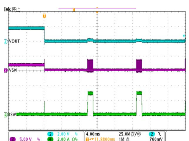
VIN=3.6V, VO=1.8V, EN=3.6V VOUT short
